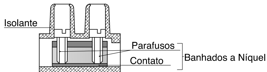
Corte AA / Esc. 1:1
