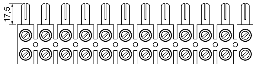
Medidas em mm / Esc. 1:2
