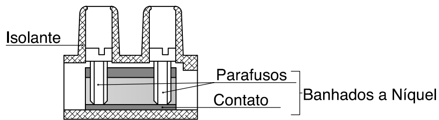
Corte AA / Esc. 1:1
