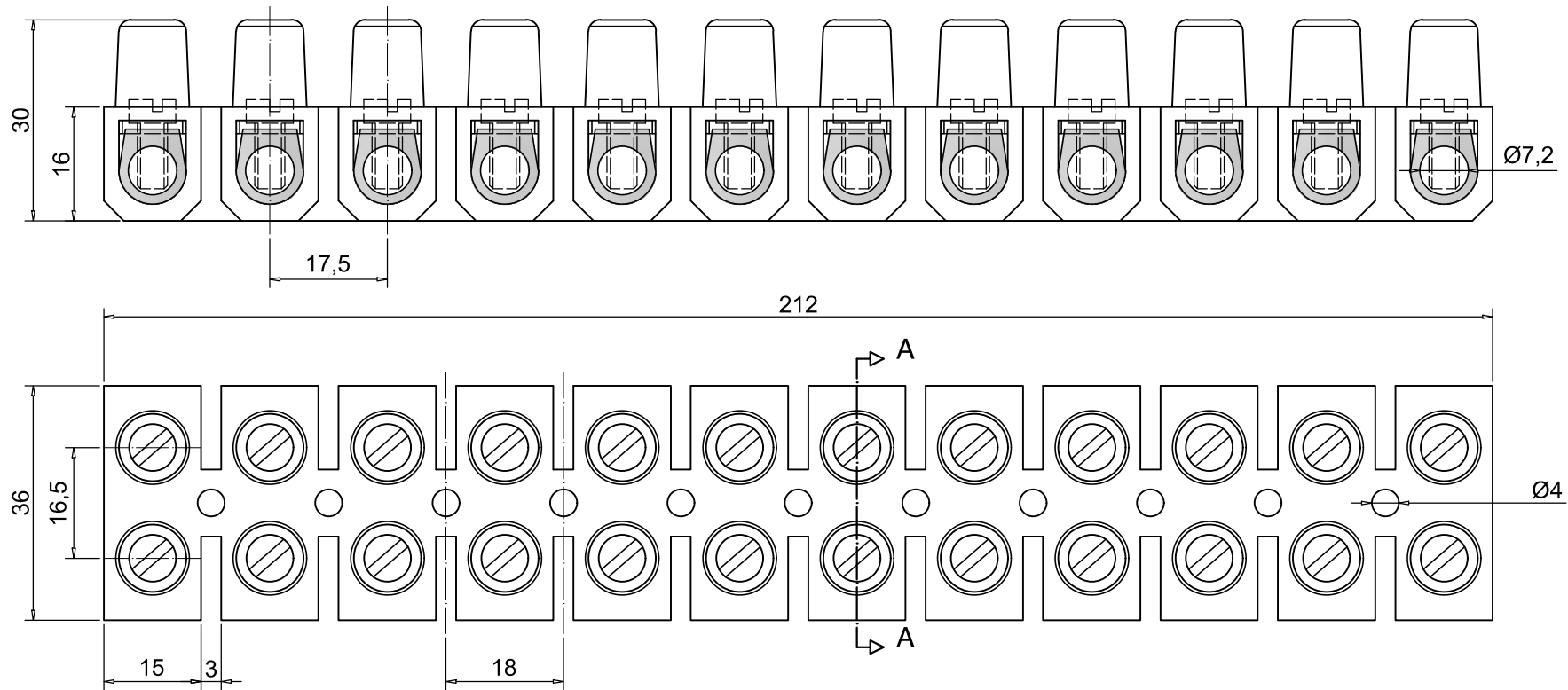
Medidas em mm / Esc. 1:1
