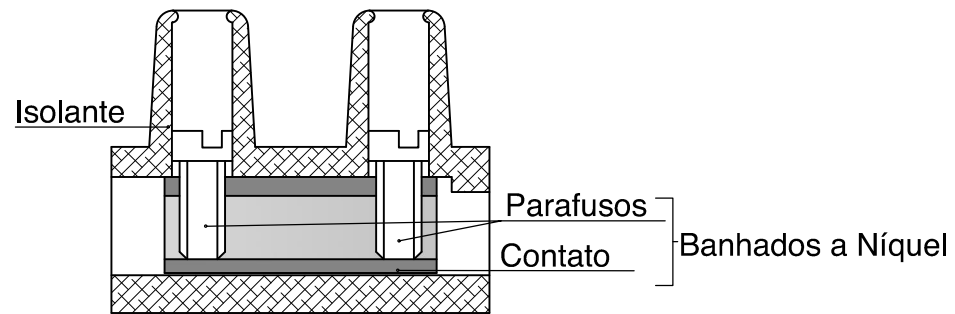
Corte AA / Esc. 2:1
