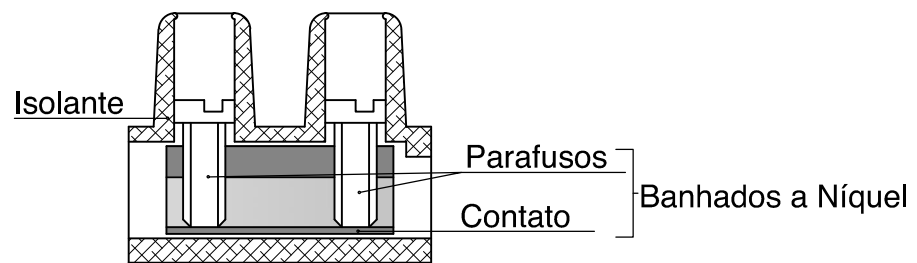
Corte AA / Esc. 2:1
