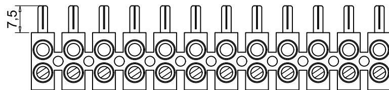
Medidas em mm / Esc. 1:1
