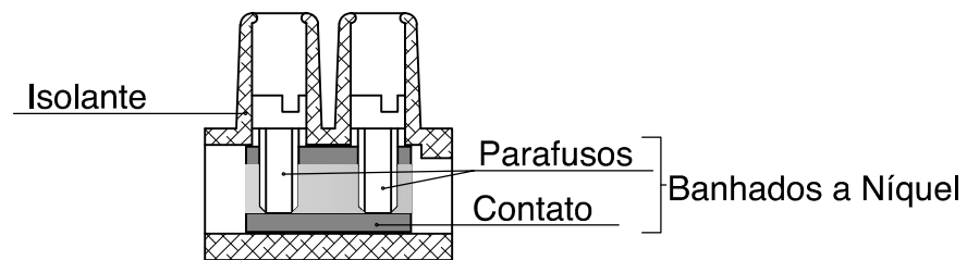
Corte AA / Esc. 2:1
