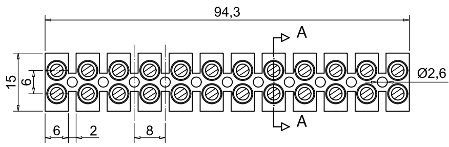
Medidas em mm / Esc. 1:1
