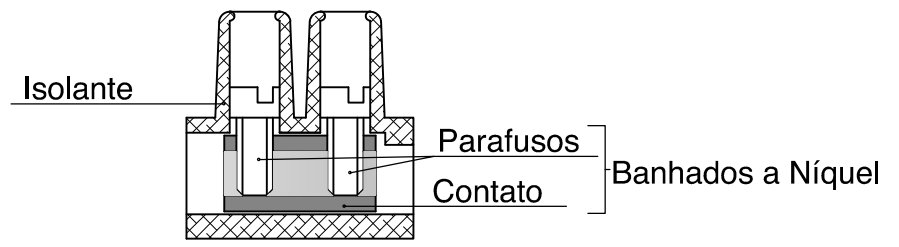
Corte AA / Esc. 2:1
