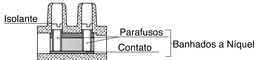
Corte AA / Esc. 1:1
