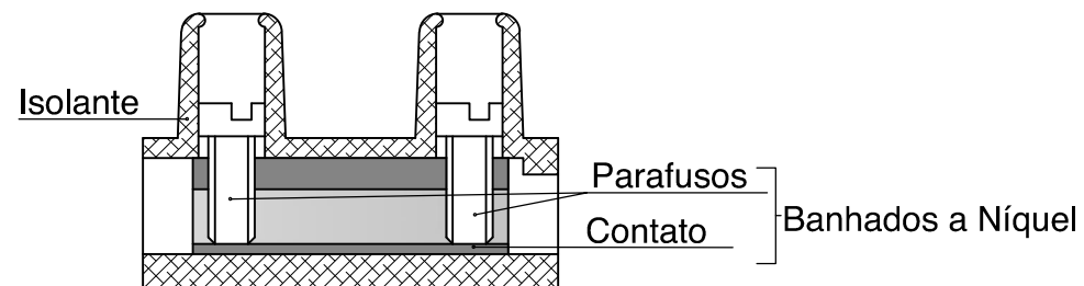
Corte AA / Esc. 2:1
