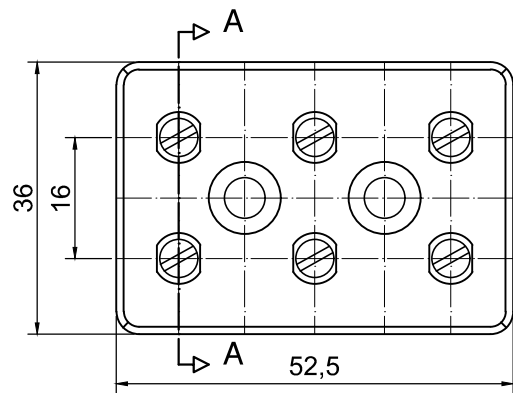
Medidas em mm / Esc. 1:1
