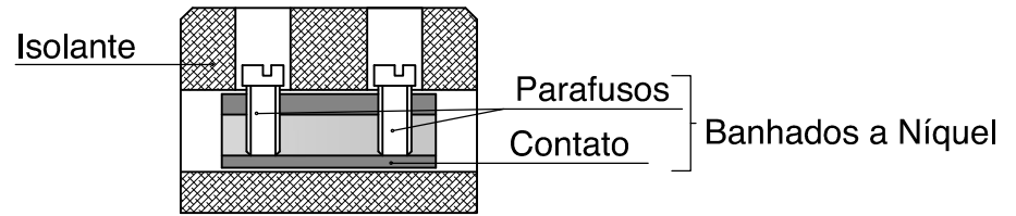
Corte AA / Esc. 1:1
