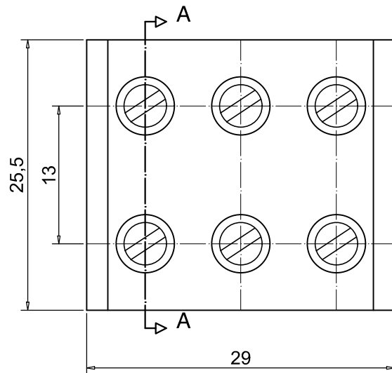
Medidas em mm / Esc. 2:1
