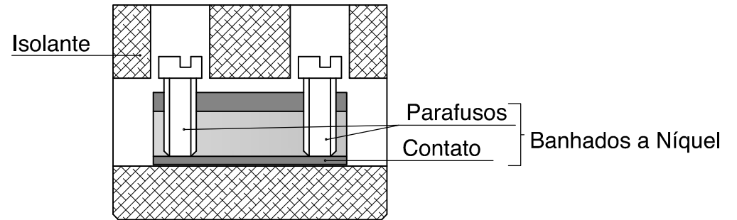
Corte AA / Esc. 2:1
