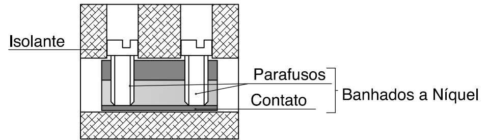
Corte AA / Esc. 2:1
