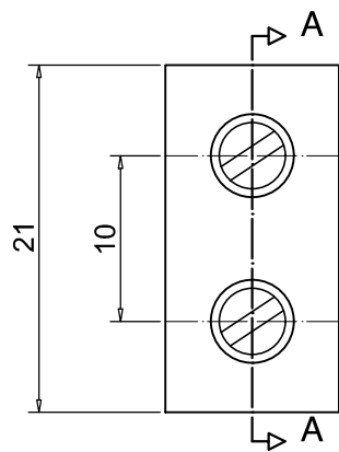
Medidas em mm / Esc. 2:1
